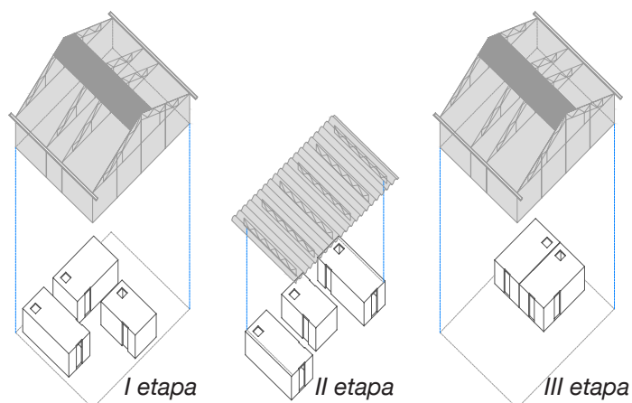
II etapa_Escola Tècnica Superior d'Arquitectura del Vallés (ETSAV), Sant Cugat del Vallés. Els mòduls van ser acopiats al mateix campus de l'escola des d'octubre 2012 fins a juny 2015.
